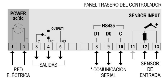
Fig. 02 – Conexiones mostradas en la etiqueta del controlador
